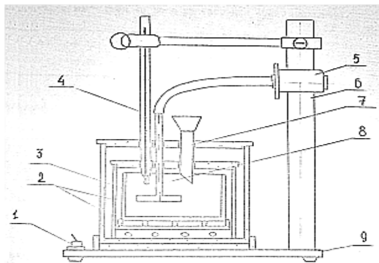
Рис. 1. Схема калориметра:
